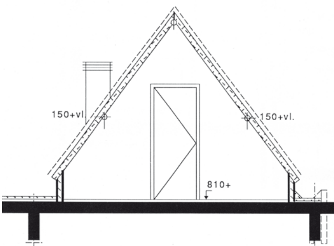
Doorsnede
